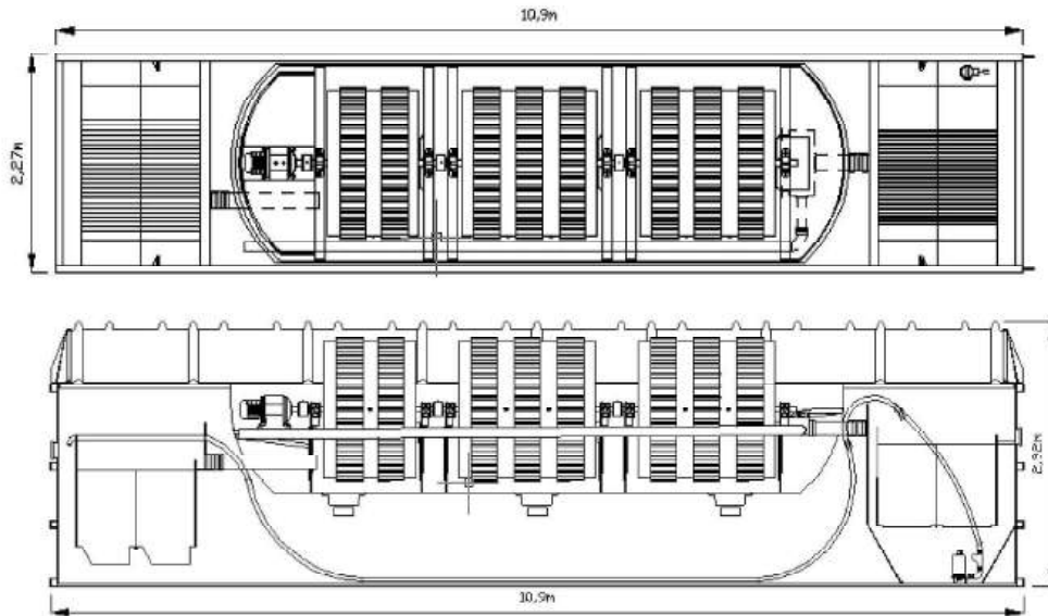
Vues en plan et en coupe d'une station BLIVET 500EH
