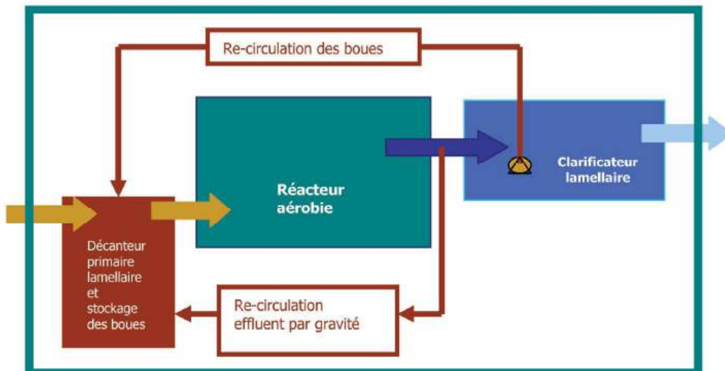
Schéma de principe de fonctionnement station BLIVET
