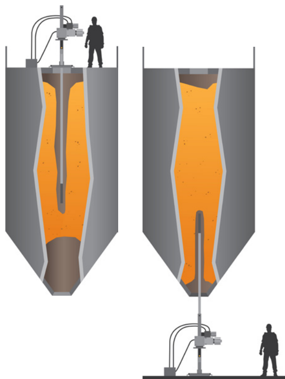
PERÇAGE PAR LE HAUT
