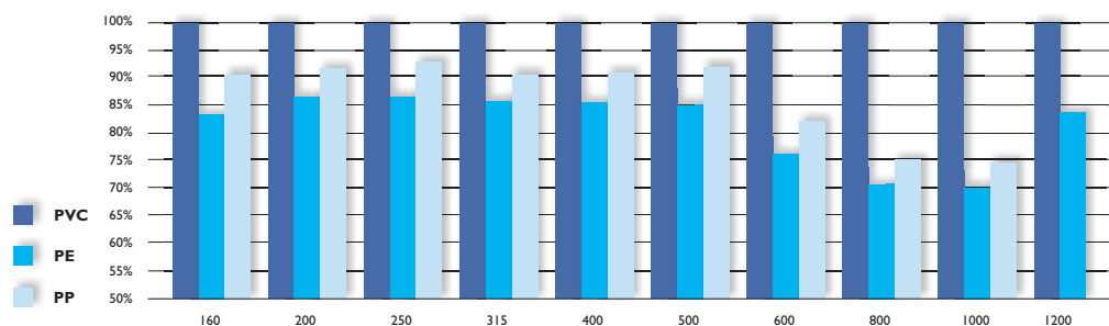
DIFERENCIAS DE CAUDAL MEDIO EN PORCENTAJE DE TUBERÍAS CORRUGADAS SN8 (BASE 100% PARA EL TUBO SANECOR®)
