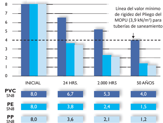
EVOLUCIÓN DE LA RIGIDEZ RCE = (E c )/D m ³ CON EL TIEMPO SEGÚN LA NORMA DIN 16961
