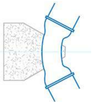
▲ Ancrages sur changements de direction
